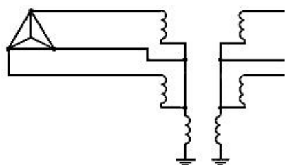
Рисунок Б.3 - Схема включения однофазных заземляемых и заземляемых двухобмоточных трансформаторов в трехфазных электрических сетях с изолированной нейтралью и напряжением 3-35 кВ
