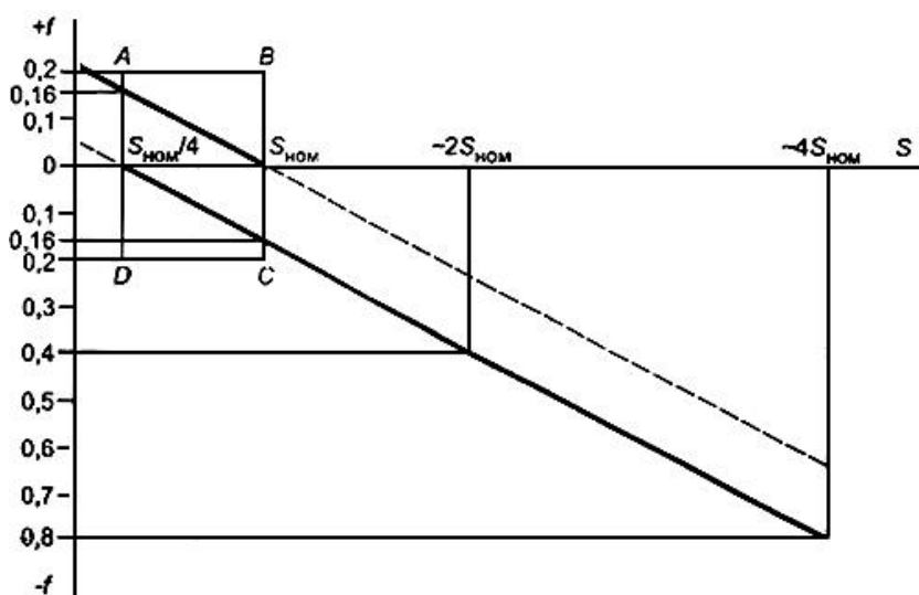
Рисунок А.1. Рекомендуемые характеристики процентного изменения вторичного напряжения трансформатора
