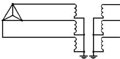
Рисунок Б.2 - Схема включения однофазных заземляемых и заземляемых двухобмоточных трансформаторов в трехфазных электрических сетях с изолированной нейтралью и напряжением 3-35 кВ
