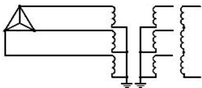
Рисунок Б.2 - Схема включения однофазных заземляемых и заземляемых двухобмоточных трансформаторов в трехфазных электрических сетях с изолированной нейтралью и напряжением 3-35 кВ
