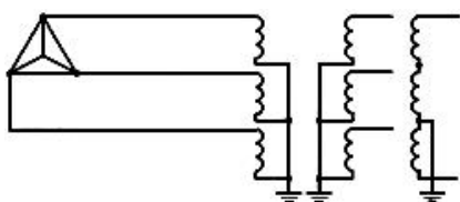
Рисунок Б.6 - Схема включения однофазных заземляемых и заземляемых двухобмоточных трансформаторов с двумя основными вторичными обмотками в трехфазных электрических сетях с изолированной нейтралью и напряжением 3-35 кВ
